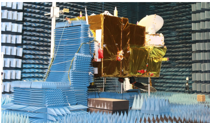
EMC试验
