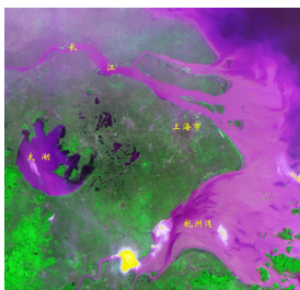
HY-1A卫星CCD成像仪长 江三角洲遥感影像图
