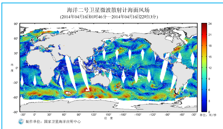
HY-2 卫星扫描微波辐射计—全球海面风速专题图（单位：米/秒） （数据时间2014年04月14日00时06分—2014年04月15日00时30分）
