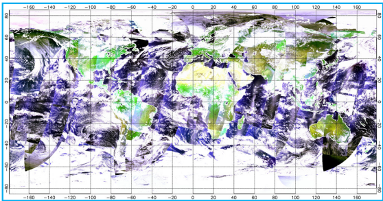
HY-1B卫星水色仪拼轨全球覆盖图
