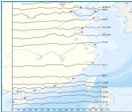
中国沿海部分验潮站海平面变化
