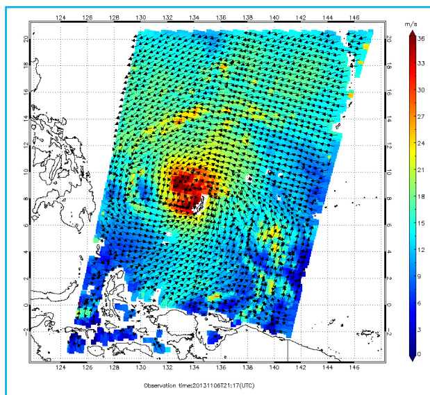
HY-2卫星微波散射计监测到的2013年第30号台风“海燕”
