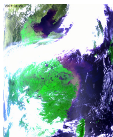
HY-1B卫星水色仪第 一轨遥感影像图
