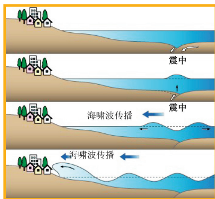
海啸发生及传播过程示意图
