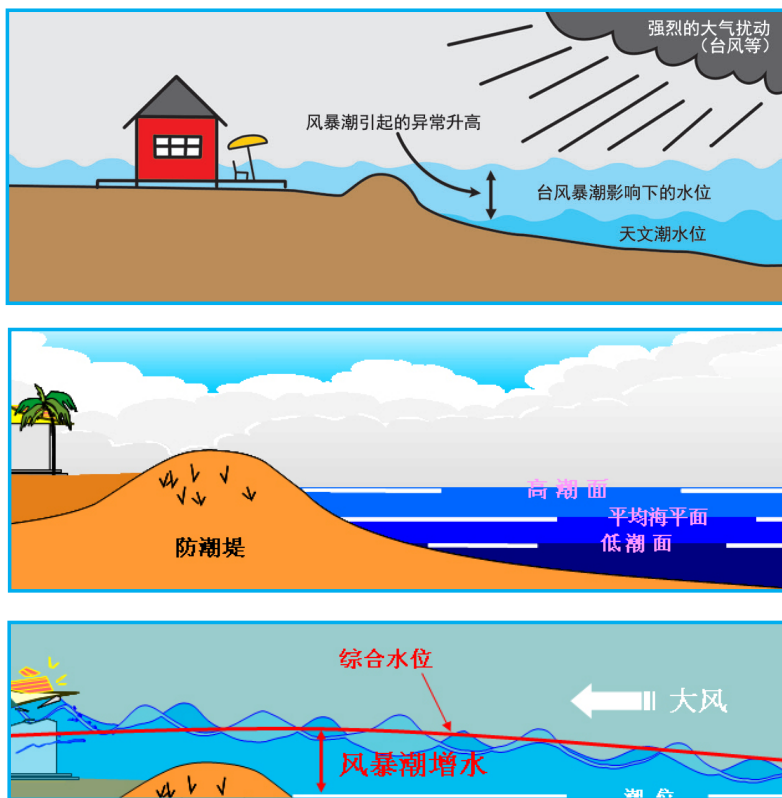
风暴潮示意图
