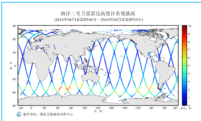
HY-2 卫星雷达高度计- 全球有效波高专题图（单位：米） (数据时间2014年04月14日23时40分—2014年04月15日23时53分)
