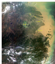
HY-1B卫星CZI成像仪 第一轨遥感影像图
