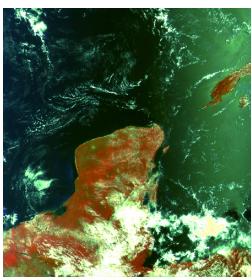
HY-1A卫星水色仪境外第 一幅图像（墨西哥湾）
