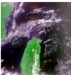
HY-1A卫星CCD成像仪 第一幅图像（台湾岛）
