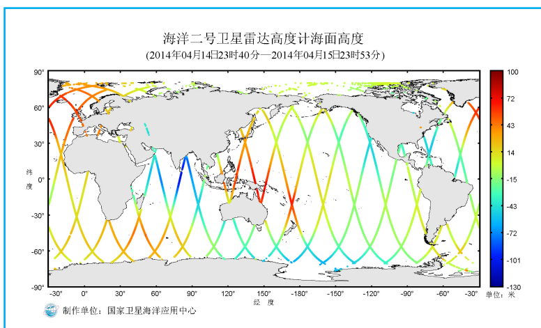
HY-2 卫星雷达高度计- 全球海面高度专题图（单位：米） (数据时间2014年04月14日23时40分—2014年04月15日23时53分)
