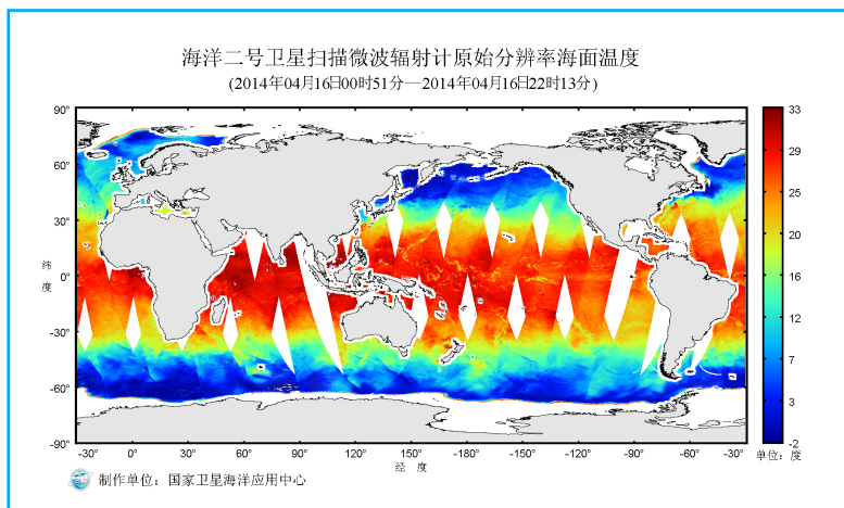
HY-2 卫星扫描微波辐射计- 全球海面温度专题图（单位：度） （数据时间2014年04月16日00时51分—2014年04月16日22时13分）
