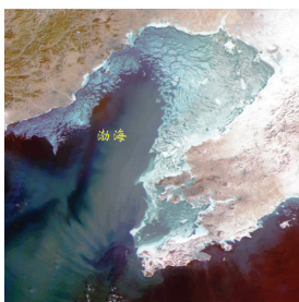
HY-1A卫星CCD成像仪渤 海海冰遥感影像图
