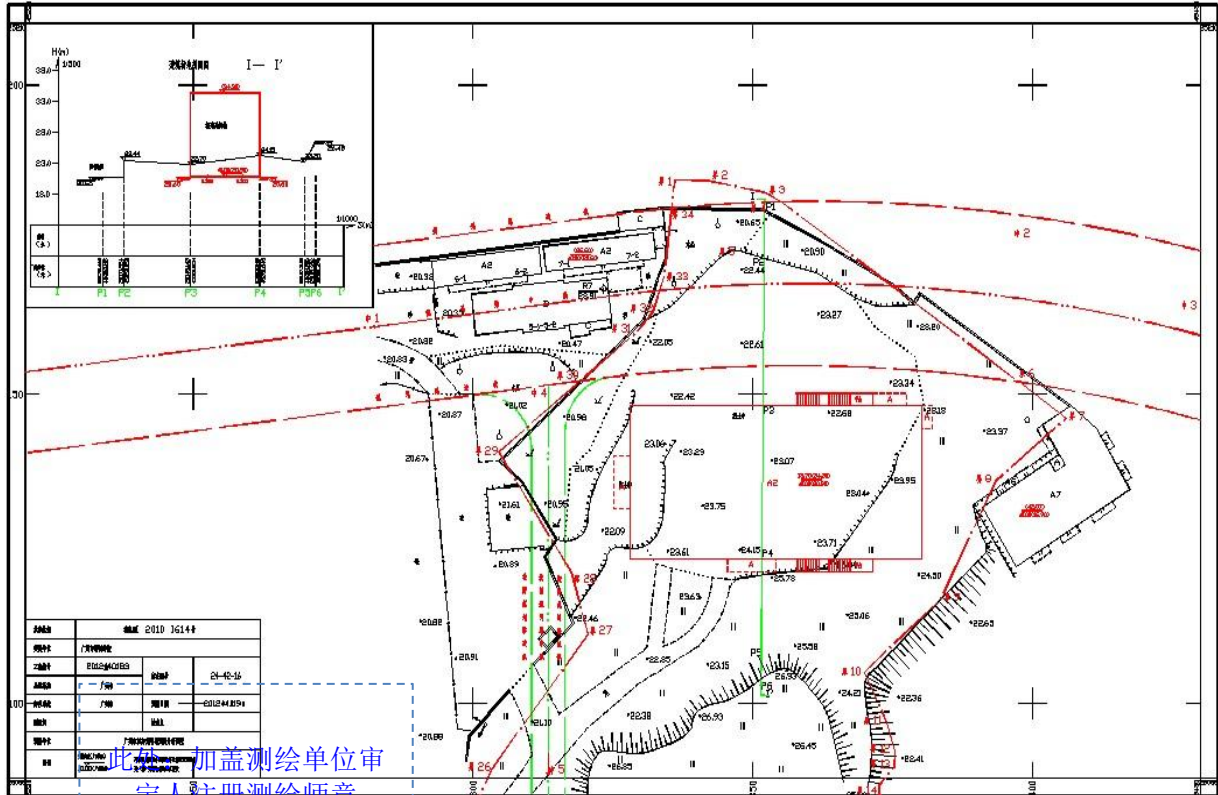
建筑场地现状地形图
