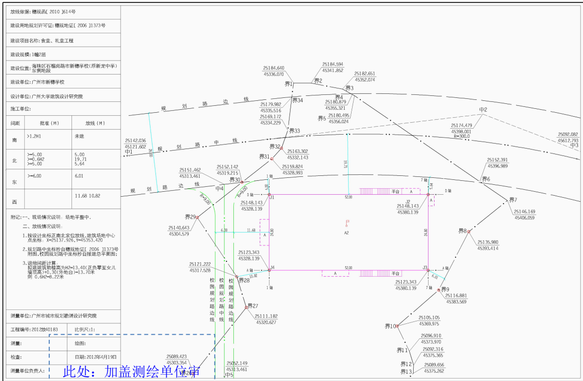
放线平面位置关系图
