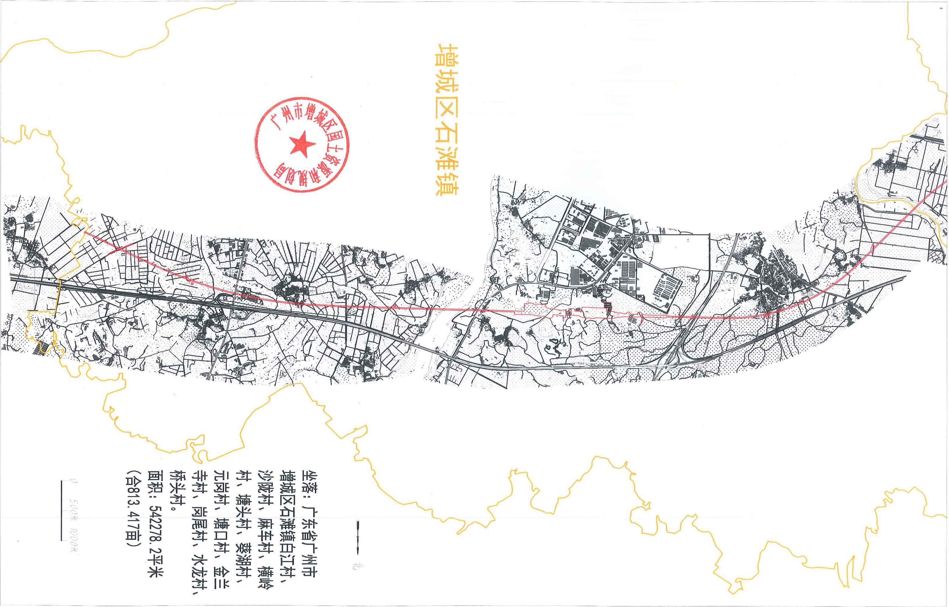
新建广州(新)塘至汕尾铁路工程项目增城境内石滩段征地示意图
