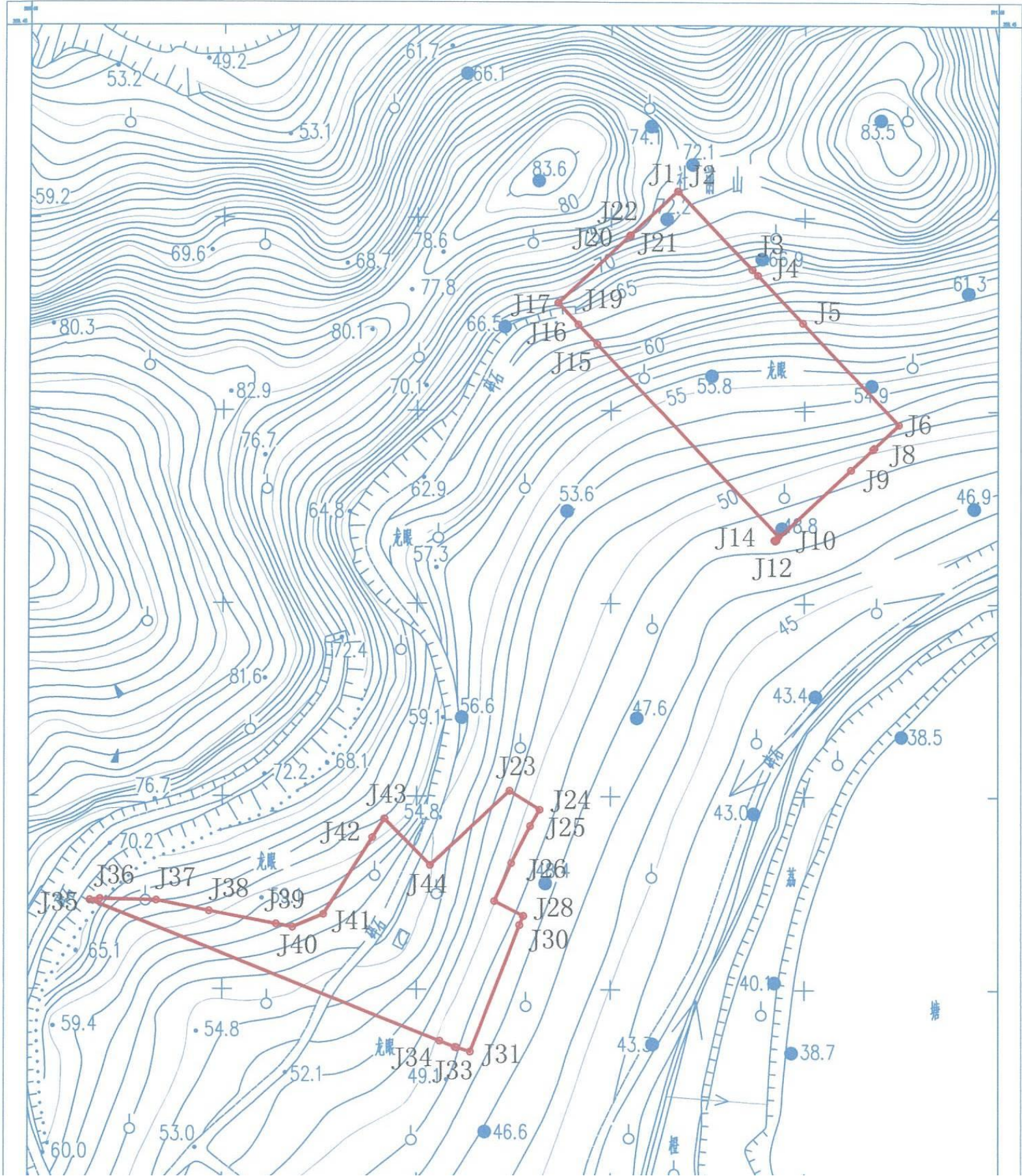
用地界址图
